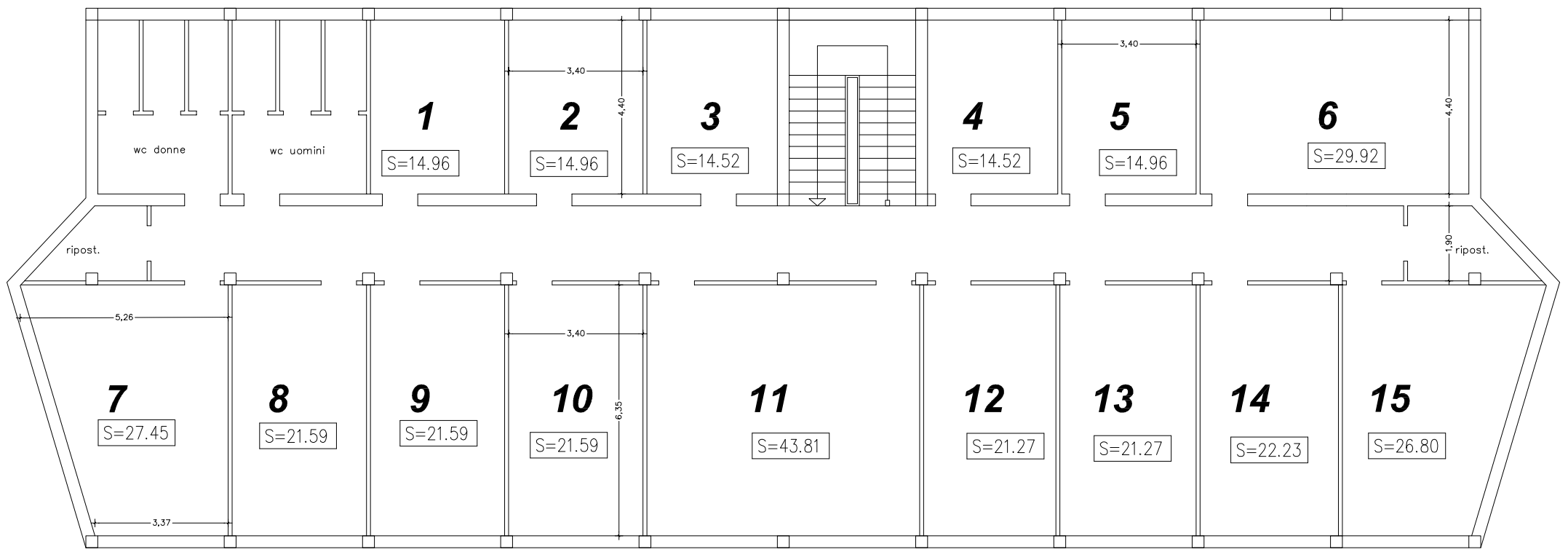
PIANO SECONDO
