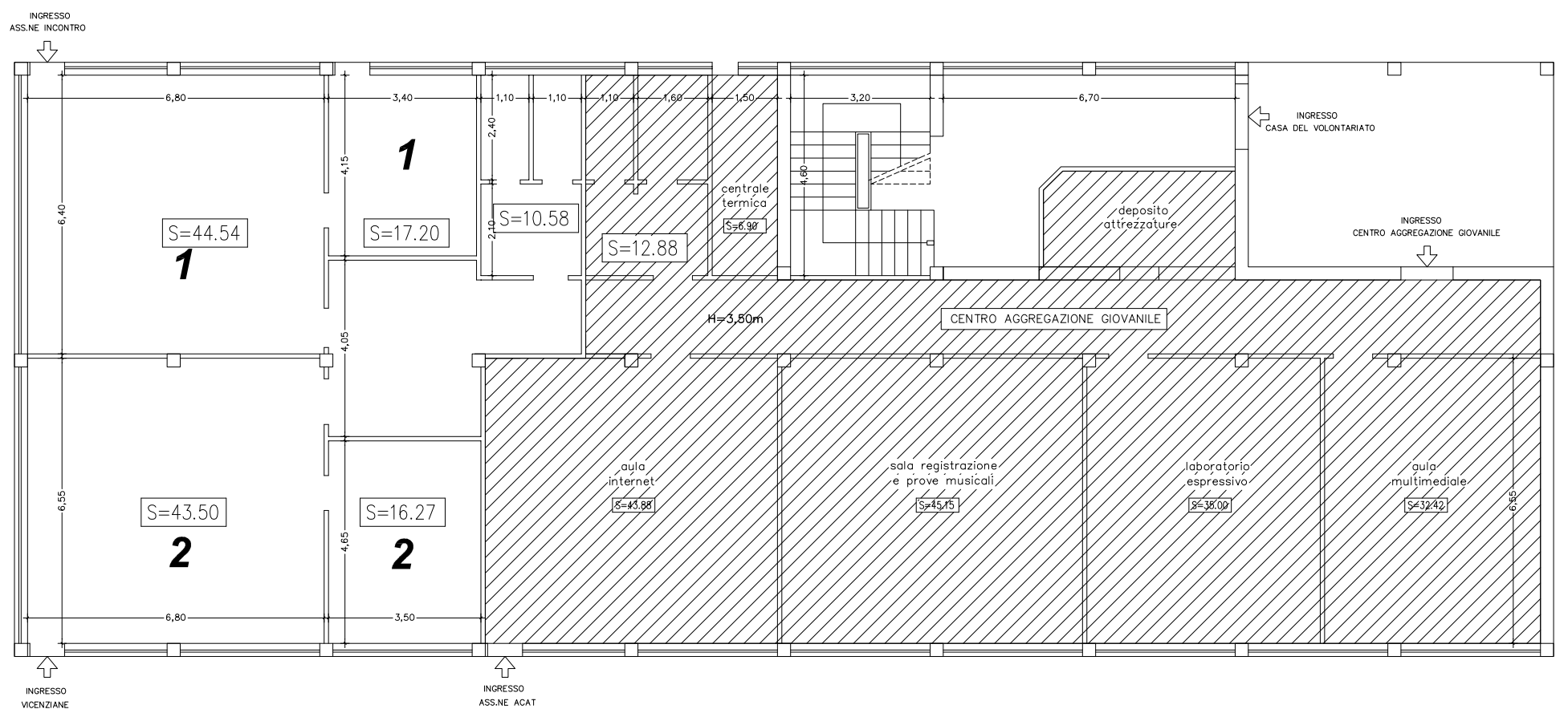
PIANO TERRA MODIFICATO
